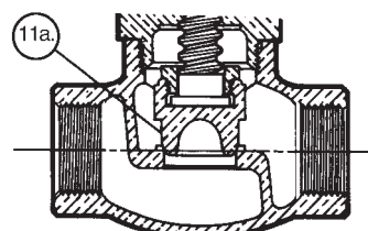
T-211-B
