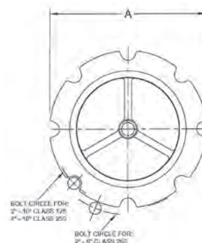
W-910-B-LF/W-960-B-LF W-910-SS/W-960-SS
