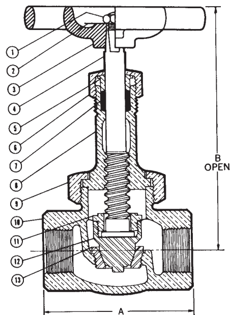
T-276-AP
