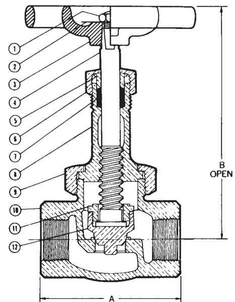
T-275-B
