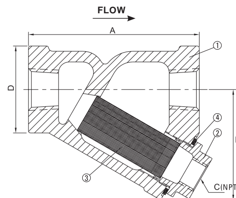
T-751-A Threaded
