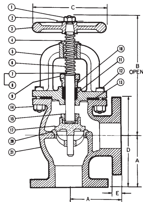
F-818-B
