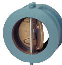
W-920-W-LF Wafer
