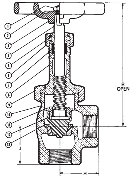
T-376-AP
