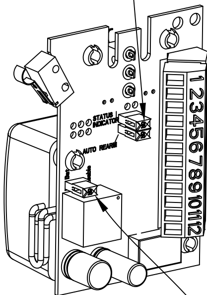
Detalles de Selectores Deslizantes
