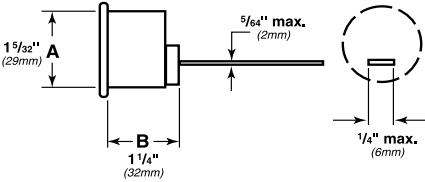
Rim — 3216 (Schlage 20-022 cam)
