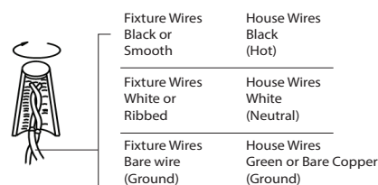
Fig. 2 Wiring
